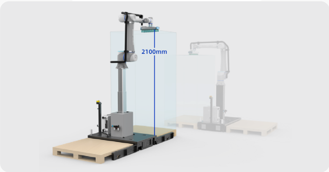
Bereik met hefkolom: Maximaal 2.100 mm
